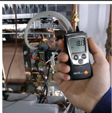
MANOMETRO
