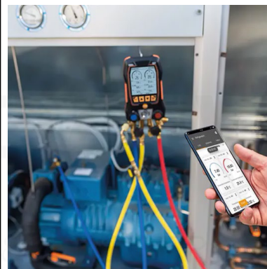
MANOMETRO REFRIGERANTE
