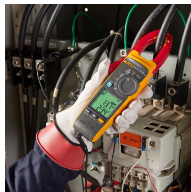
AMPERIMETRO
