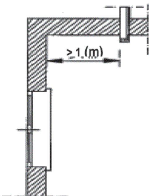
Figura 48. Distancia de Sombrero a Pared Lateral con Ventana o Ventilación.
