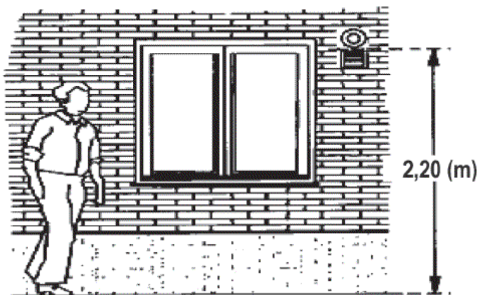
Figura 43. Altura mínima de sombrerete de artefacto.
